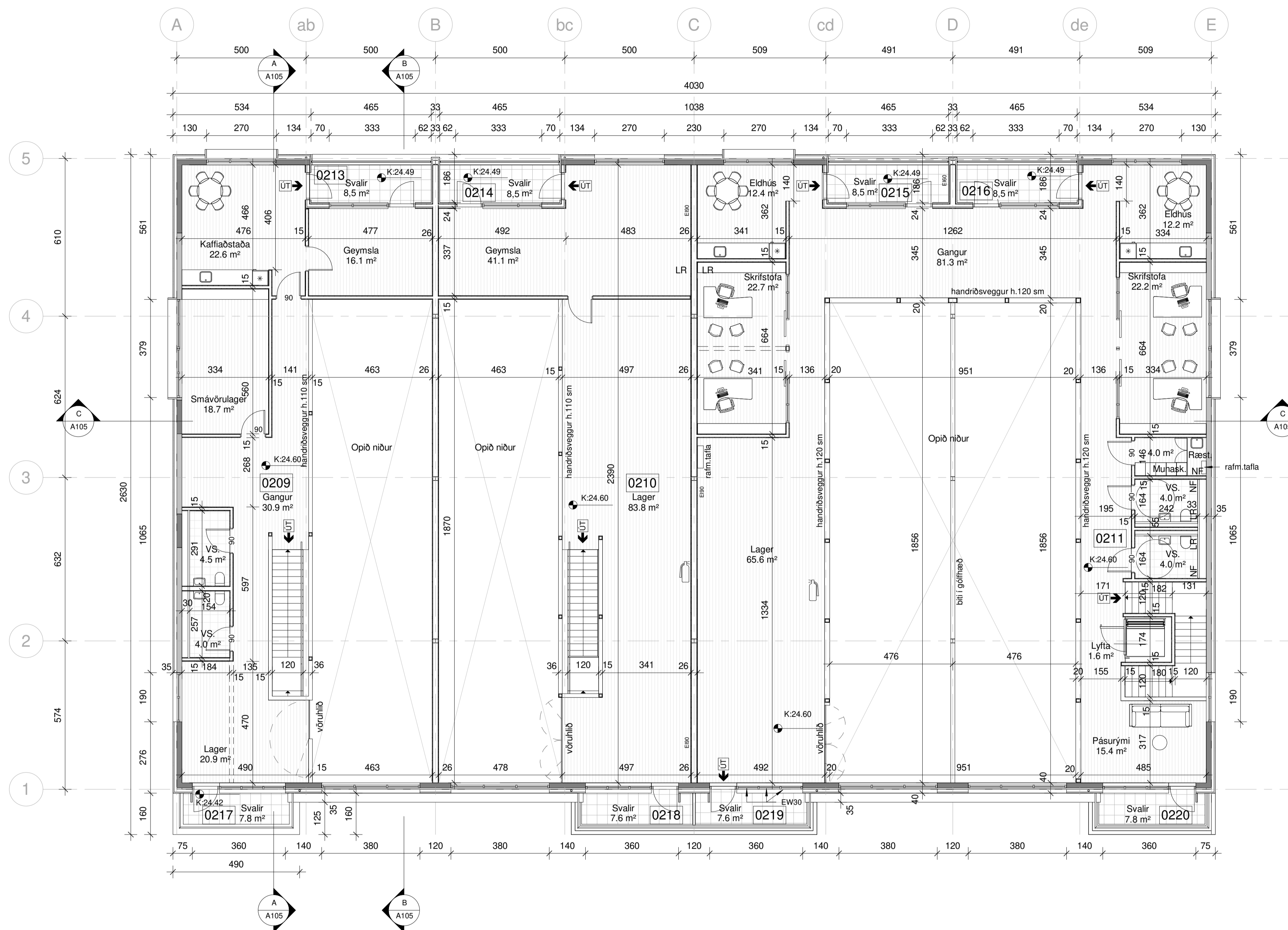
2. hæð, millifletir 1 : 100
