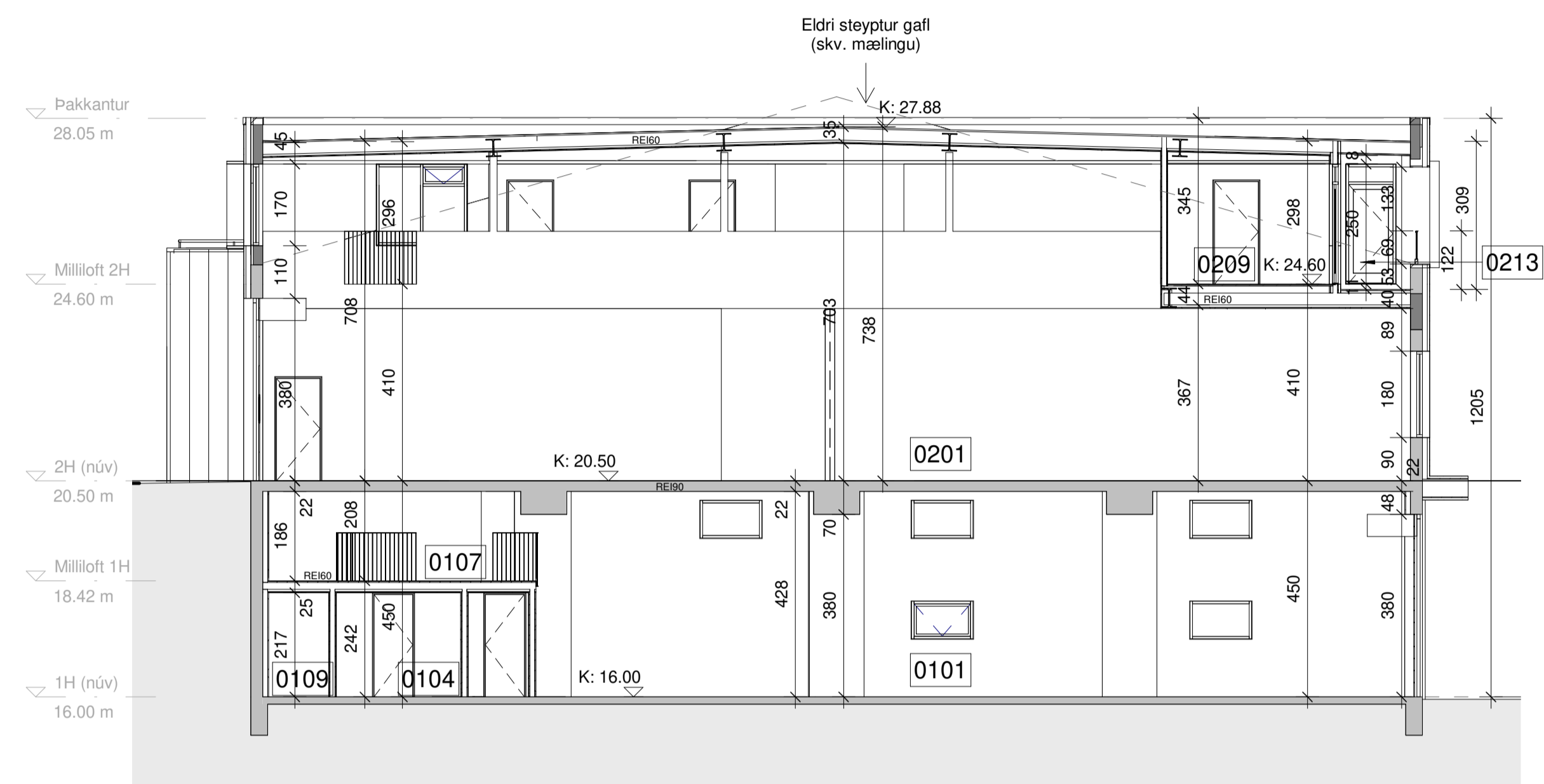
Snið B-B 1 : 100
