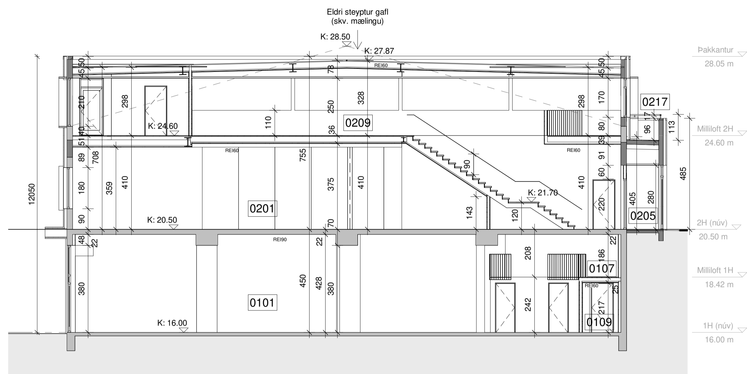
Snið A-A 1 : 100
