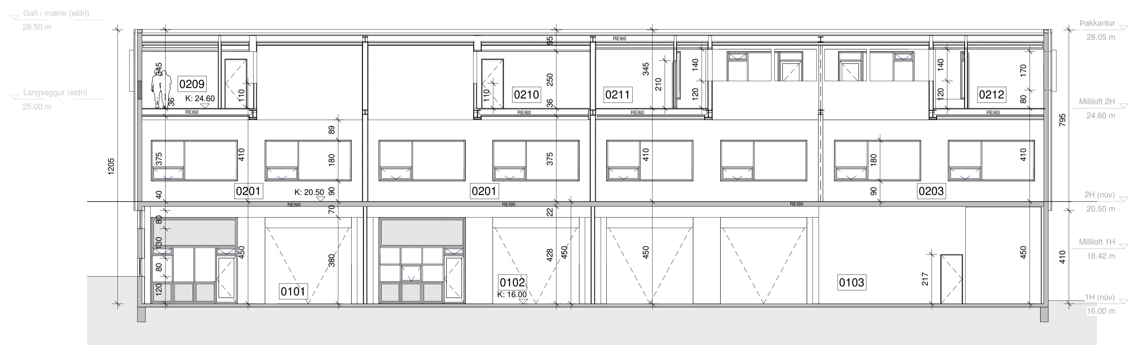
Snið C-C 1 : 100
